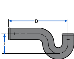
LONG P-TRAP
